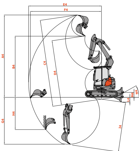
Verlängerter Ausleger (2.110 mm)
